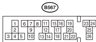
继电器支架
